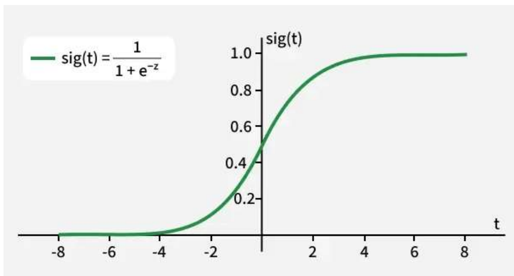
Sigmoid function
